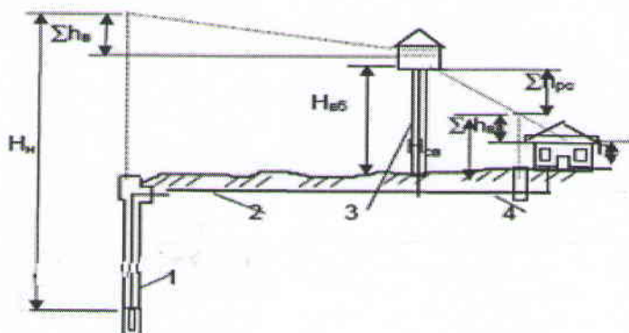
Рис. 1 - Структура системы водоснабжения сельского поселения Узюково.
